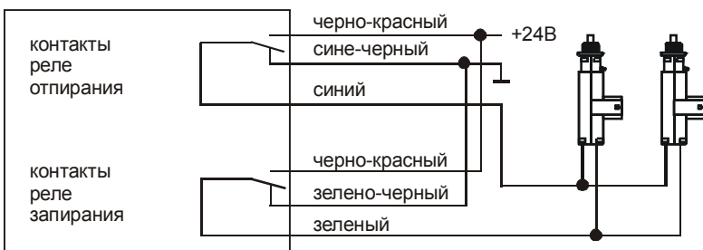
Схема подключения к пневматической системе запирания
