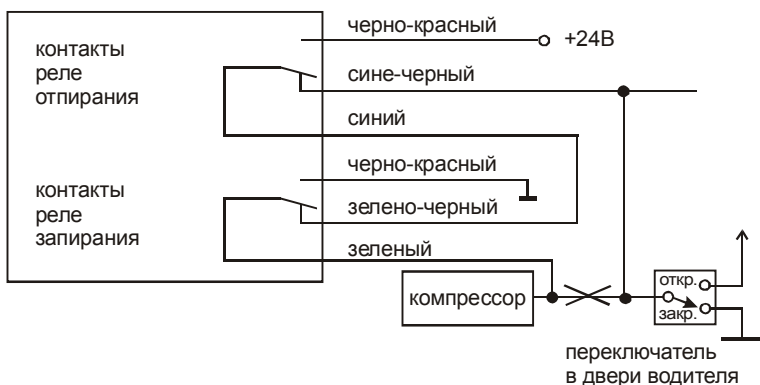
Схема подключения к пневматической системе запирания
