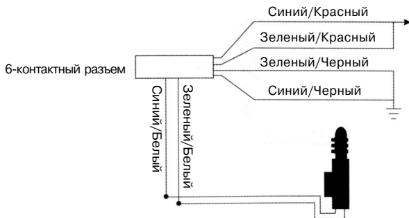
Схема 6. Установка дополнительных электроприводов
