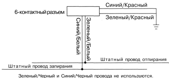
Схема 1. 3-проводная система с отрицательной полярностью (большинство японских автомобилей)
